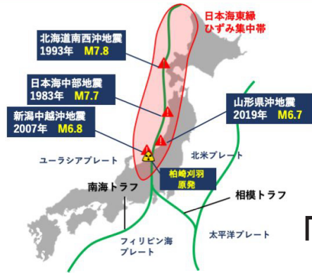
日本海東縁ひずみ集中帯とその付近で起きた主な地震
